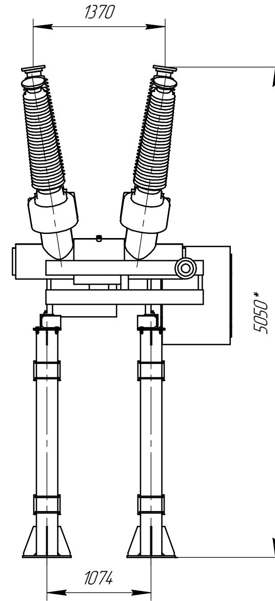
Блок выключателя БО.110.ВК(Б)/ХХ*/14,5-ХХХ**
